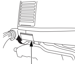
DZINĒJA PĀRSEGA FIKSATORS
