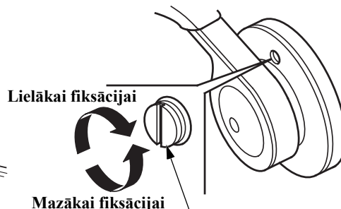
VADĪBAS SVIRAS FIKSĀCIJAS REGULATORS
