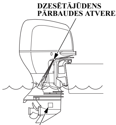
DZESĒTĀJŪDENS IEPLŪDES ATVERE (katrā pusē)
