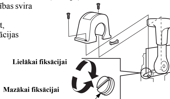
VADĪBAS SVIRAS FIKSĀCIJAS REGULATORS
